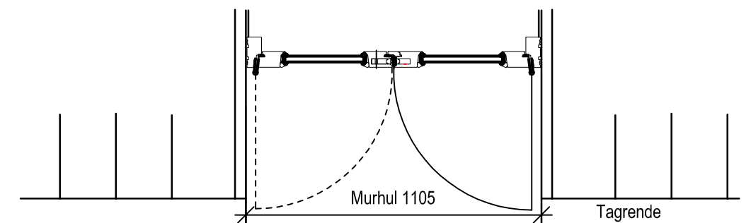
Altandør fra værelse/køkken. 1:20
