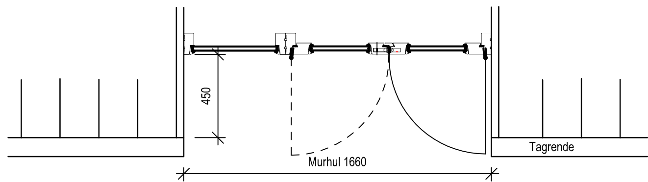
Altandør fra værelse, 5. sal 1:20
